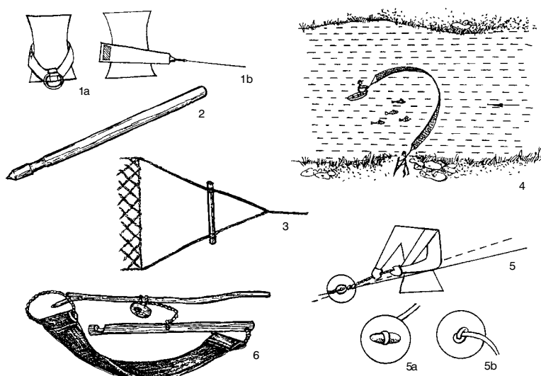
1 pav.* Žvejyba traukiamuoju tinklu: 1 – tinklas stabdomas pastojikės diržu: a – vaizdas iš priekio, b – vaizdas iš šono. Jurbarko r., Viešvilė; 2 – artuolis. Šilutės r., Girininkų k.; 3 – brankas. Šilutės r., Girininkų k.; 4 – tinklo užmetimo schema; 5 – traukimas plėškėmis (a, b – sagutė tinklui pagauti, vaizdas iš abiejų pusių). Jurbarko r., Viešvilė; 6 – juosta tinklui traukti. Nidos istorijos muziejus
