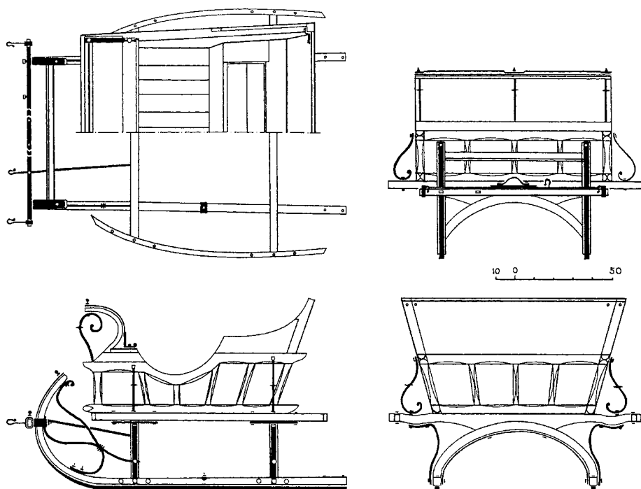
13 pav. Rogutės (projekcijos). Šakių r. Karališkių k. IIES 635/56b. 1975 m. Piešė M. Puzinaitė
