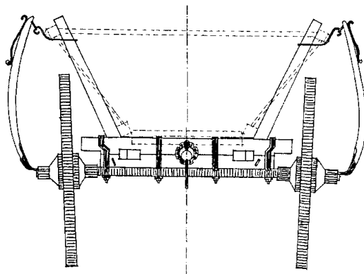
2 pav. Porinio briko užpakaliniai ratai su lušnimis ir lušnapančiais. XX a. 3-iasis dešimtmetis. Šilalės r., Lembo k. M. Puzinaitės brėž. 1973 m.
