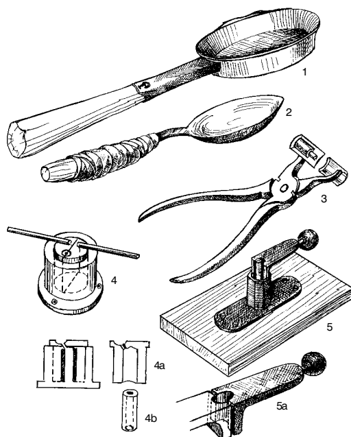
12 pav. Priemonės švininiams svoreliams lieti: 1, 2 – indelis švinui lydyti ir šaukštas jam pilti. Šakių r., Kidulių k.; 3 – replės. Kauno r., Vilkija; 4 – mašinka (a – pjūvis, b – svorelis). Jurbarko r., Molynės k.; 5 – mašinka (a – abi rankenos ištrauktos). Šakių r., Kidulių k.
