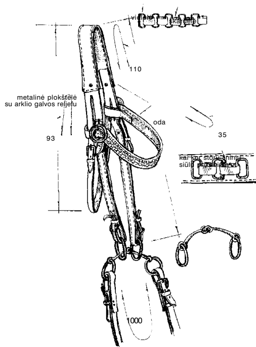
23 pav. Kamanos. Šilalės r., Paragaudžio k. 2001 m. R. Butvilienės pieš.
