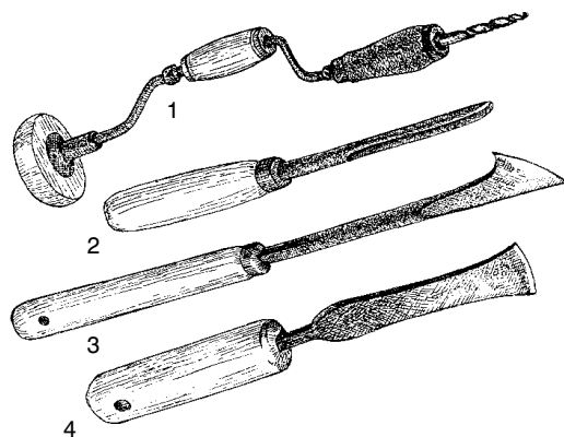
24 pav. Račiaus įrankiai: 1 – vinda; 2 – kaltas; 3 – kaltas tekinti, pjaustyti; 4 – kaltas. Kvėdarna. 2001 m. R. Butvilienės pieš.
