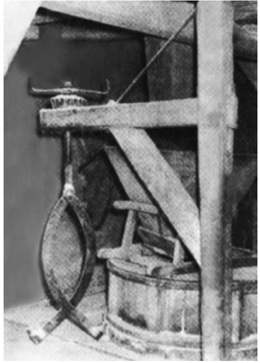
35 pav. Grimzdų malūno girklys
