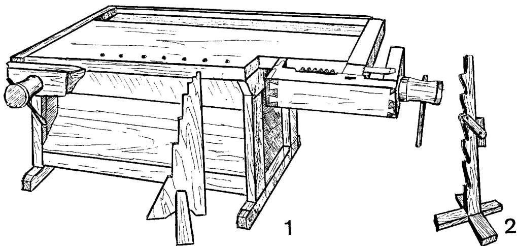
22 pav. 1 – varstotas. XX a. 4 dešimtmetis. Šakių r. Gelgaudiškis. IIES 1269/69; 2 – atrama (tarnas, berniukas) prie varstoto. XX a. 4 dešimtmetis. Šakių r. Lekėčiai. IIES 1269/71. 1988 m. Piešė G. Griška
