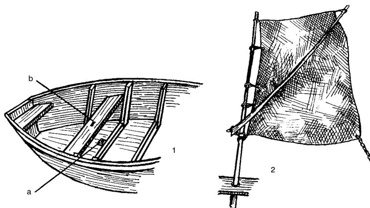
21 pav. Burinė valtis. Jurbarko r., Veliuona; 1a – trinkelė burės stiebui; 1b – skylė stiebui sėdynėje; 2 – burė
