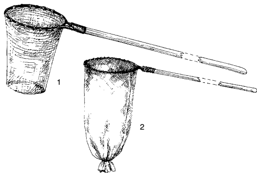
2 pav. Samčiai: 1 – stintoms gaudyti. Jurbarko r., Viešvilės k.; 2 – žuvis iš traukiamojo tinklo senti. Šilutės r., Paleičių k.
