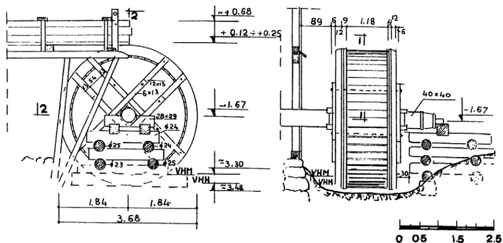
14 pav. Gražjūrio vandens malūno rato schema
