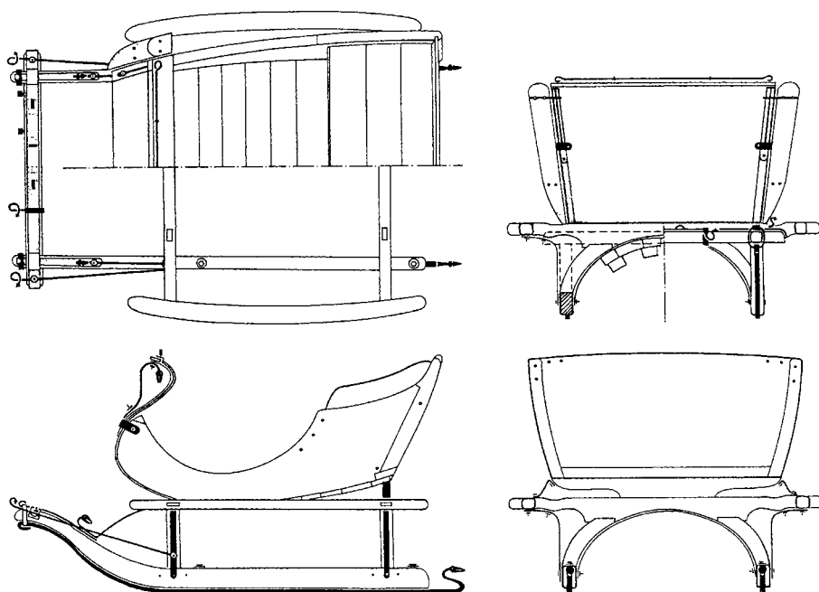
12 pav. Rogės (projekcijos). 1930 m. Šakių r. Plynių k. IIES 635/56. 1975 m. Piešė M. Puzinaitė
