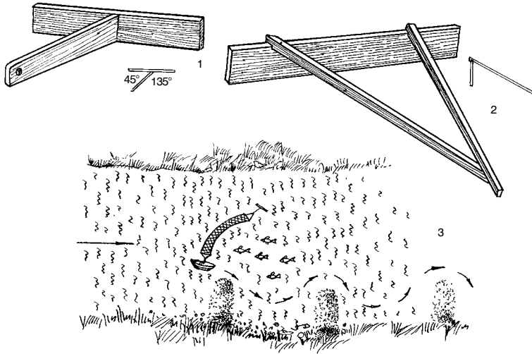
4 pav. Plūdurai: 1, 2 – Kauno r., Vilkija; 3 - tinklaičio plukdymo schema
