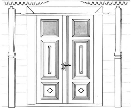
20 pav. Prieangis. V. Endriukaičio sodyba, Leliokiškės k. J. Jasinskaitės pieš.
