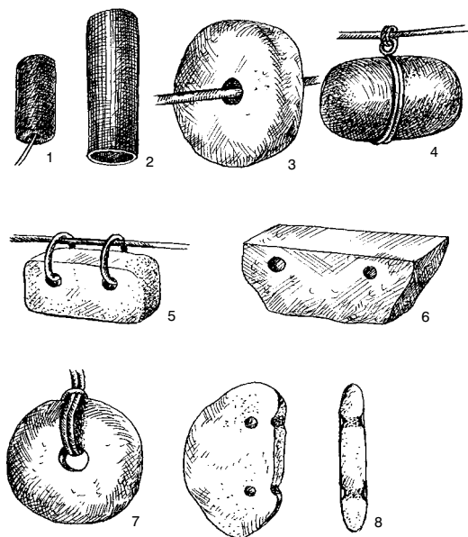
11 pav. Svoreliai. Kauno r., Vilkija. 1 – švininis; 2 – metalinis vamzdelis; 3, 7 – cementiniai; 4 – akmeninis; 5, 6, 8 – cementiniai traukiamajam tinklui
