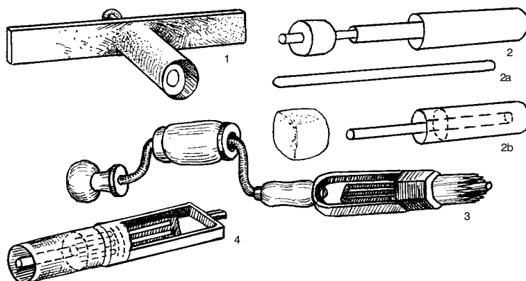
10 pav. Prietaisai plūdėms daryti: 1 – plūdei iš putplasčio išpjauti. Jurbarko r., Viešvilės k.; 2 – skylei plūdeje išpjauti (b), išpjautam gabaliukui išstumti (a). Jurbarko r., Viešvilės k.; 3 – ranka sukamas prietaisas. Šakių r., Kidulių k.; 4 – elektra sukamas prietaisas. Jurbarko r., Molynės k.
