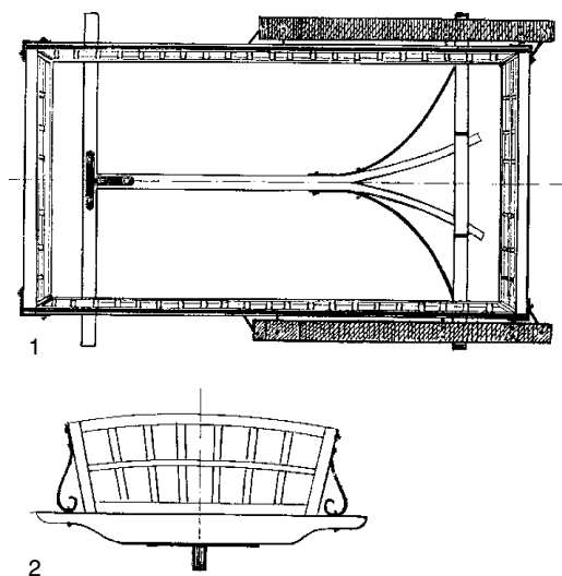
5 pav. 1 – brikelio, gaminto XX a. 4 dešimtm., projekcija iš viršaus. Šilalės r., Padievyčio apyl. M. Puzinaitės brėž. 1973 m.; 2 – brikelio užgalis. XX a. 4 dešimtm. M. Puzinaitės brėž. 1973 m.
