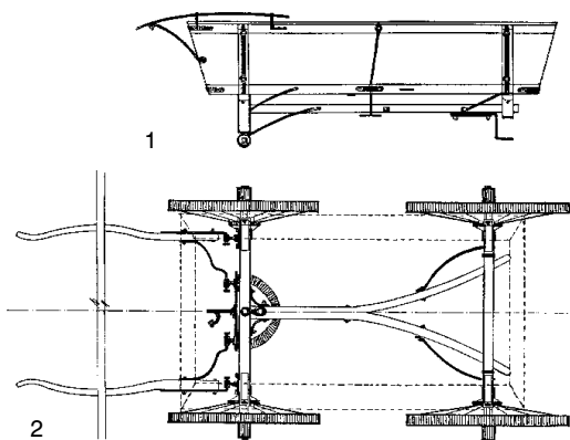
4 pav. 1 – brikelio, gaminto 1925 m., viršutinės dalies projekcija iš šono. Šilalės r., Padievyčio apyl. M. Puzinaitės brėž. 1973 m.; 2 – brikelio, gaminto 1925 m., apatinė dalis. Šilalės r., Lembo k. M. Puzinaitės brėž. 1973 m.
