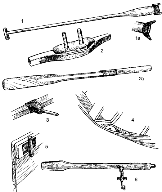
20 pav. Irklai: 1 – stumiamasis. Kauno r., Pelenių k. 1a – apkausto forma. Jurbarko r., Molyinės k.; 2 – trinkelė su pirštais įdedamajam irklui (2a – įdedamasis irklas). Veliuona; 3 – irklo metalinis pirštas. Kelmės r.; 4 – medinė trinkelė vidinėje valtys pusėje. Trakų r.; 5 – metalinis vamzdelis irklui įstatyti. Zarasų r.; 6 – irklas vamzdelinėje apkaboje. Rokiškio r.
