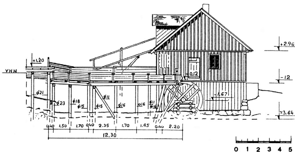
19 pav. Malūno vaizdo schema iš galo
