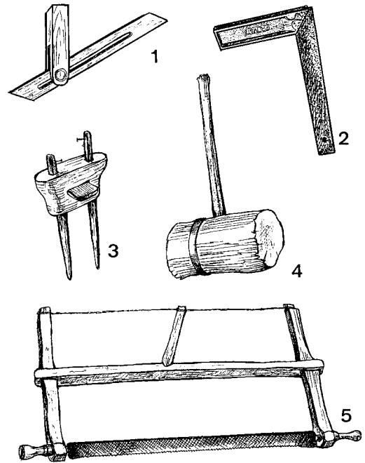
20 pav. Račiaus įrankiai: 1 – šmygė (lankstomas vinkelis). XX a. 3 dešimtme. Šakių r. Kiduliai. IIES 1269/80; 2 – vinkelis. XX a. 3 dešimtme. Šakių r. Kiduliai. IIES 1269/79; 3 – rėžtukas. XX a. 3 dešimtme. Šakių r. Slavikai. IIES 1269/82; 4 – šlėga. XX a. 4 dešimtme. Šakių r. Kriūkai. IIES 1269/76; 5 – rėminis pjūklas. XX a. 5 dešimtme. Šakių r. Slavikai. IIES 1269/72. 1988 m. Piešė G. Griška
