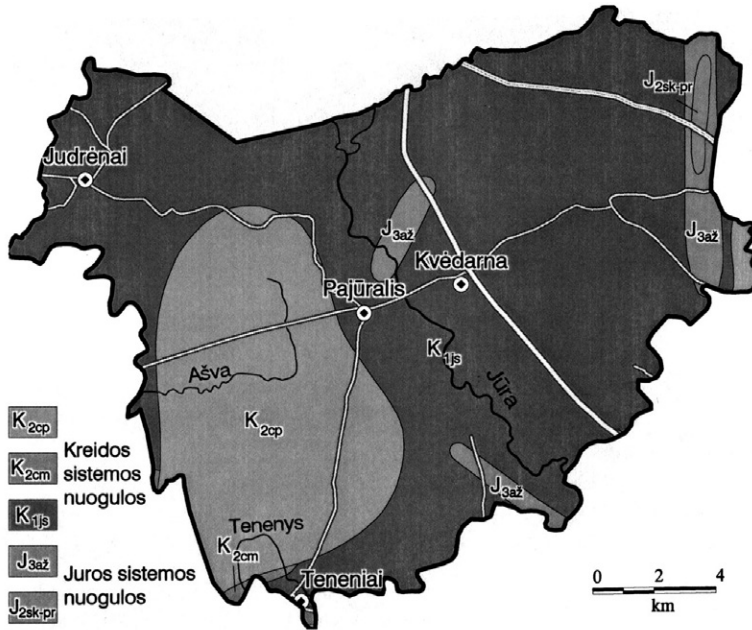
Prekvartero geologinis žemėlapis. M 1:200 000
