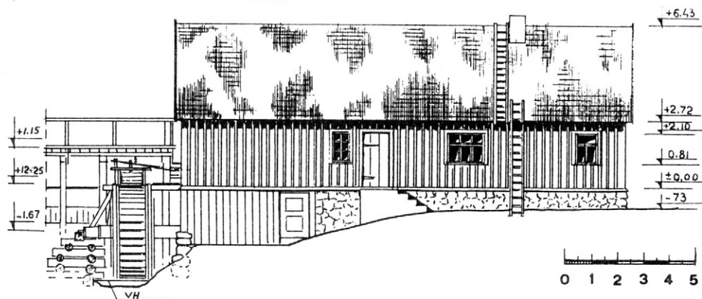
20 pav. Gražjūrio malūno vaizdo schema iš kitos namo pusės
